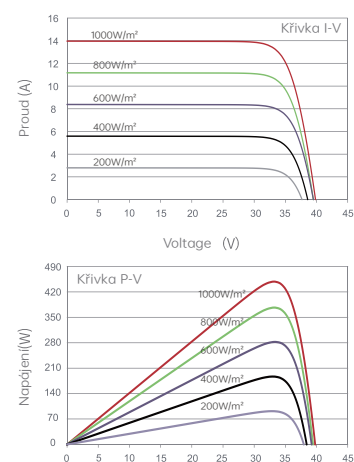
Křivky proud-napětí a výkon-napětí (430W)
